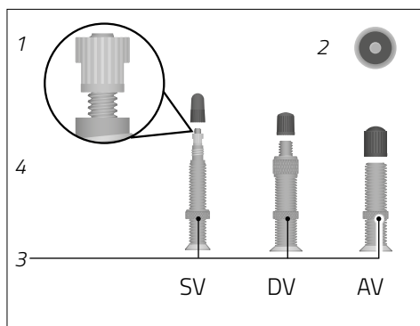
Abb.: Ventilarten (exemplarisch)
