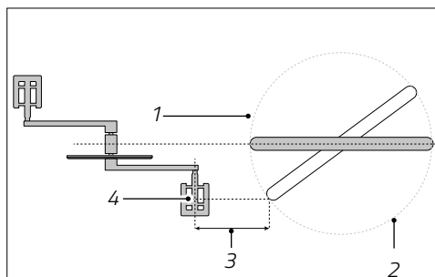
Abb.: Abstand zwischen Pedal und Vorderrad (exemplarisch)
