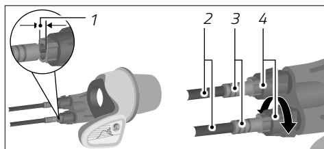
Abb.: Spiel der Schaltzughülle (links) und Einstellschraube (rechts) (exemplarisch)
