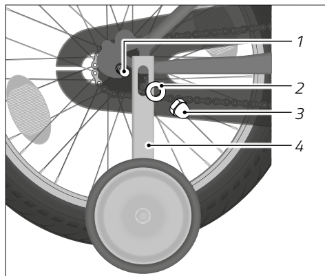
Abb.: Stützrad montieren (exemplarisch)
