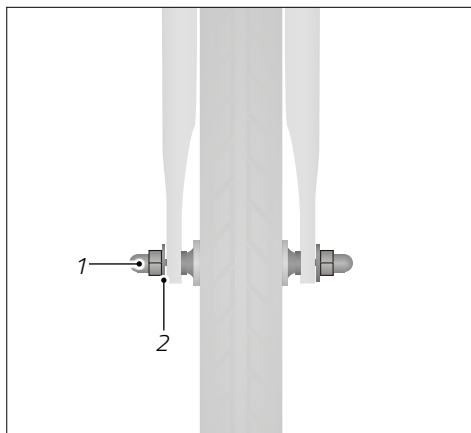
Abb.: Laufrad mit Schraubachse (exemplarisch)
