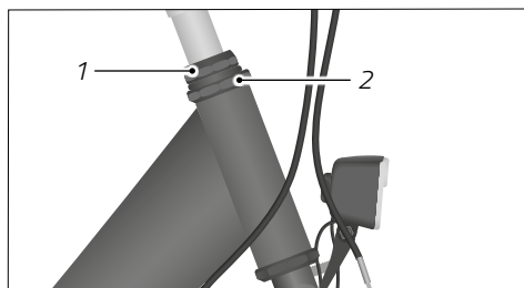
Abb.: Innenklemmung (exemplarisch)
