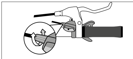
Abb.: Zugspannschraube an dem Schalthebel (exemplarisch)
