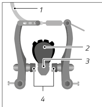
Abb.: Mechanische Felgenbremsen (exemplarisch)
