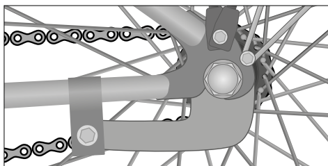
Abb.: Rücktrittbremse (exemplarisch)
