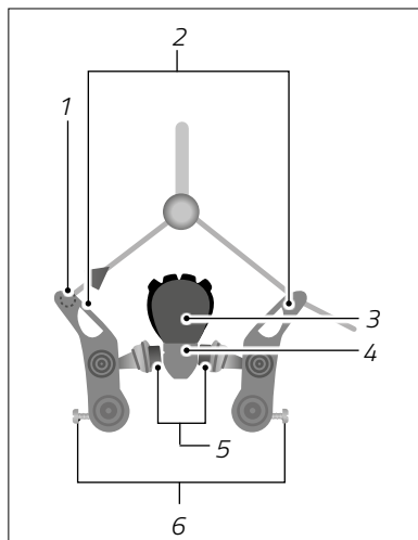
Abb.: Felgenbremse mit Seilnippel (exemplarisch)
