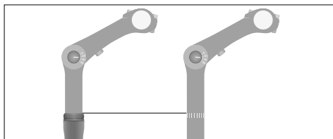
Abb.: Markierung der Mindesteinstecktiefe bei einem Schaftvorbau mit Innenklemmung (exemplarisch)
