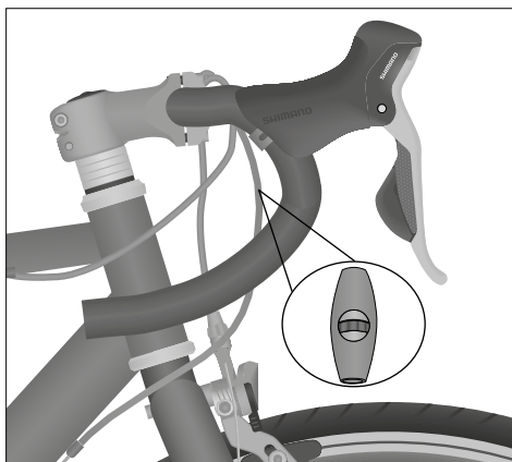
Abb.: Kettenschaltung einstellen (exemplarisch) Einstellschraube mit Verstellrad für die Zugspannung
