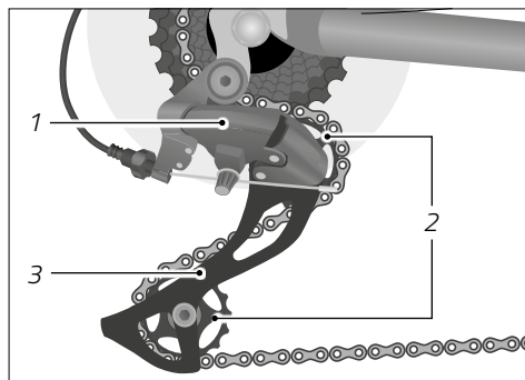
Abb.: Bewegliche Komponenten einer Kettenschaltung (exemplarisch)
