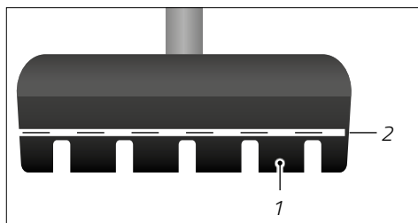
Abb.: Brems Schuh mit Verschleißindikator (exemplarisch)
